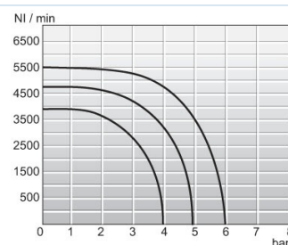
Durchflussdiagramm 1/2"
