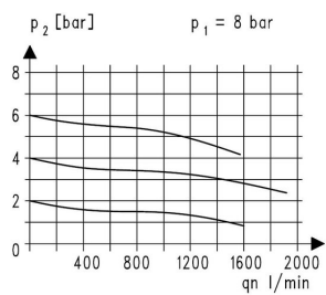
Átfolyási diagramm
