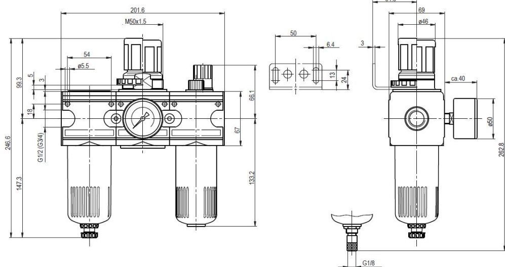
félautomata leeresztőszelő
