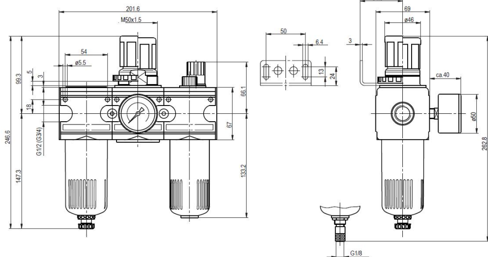
félautomata leeresztőszelep
