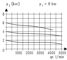
Wykres przepływu
