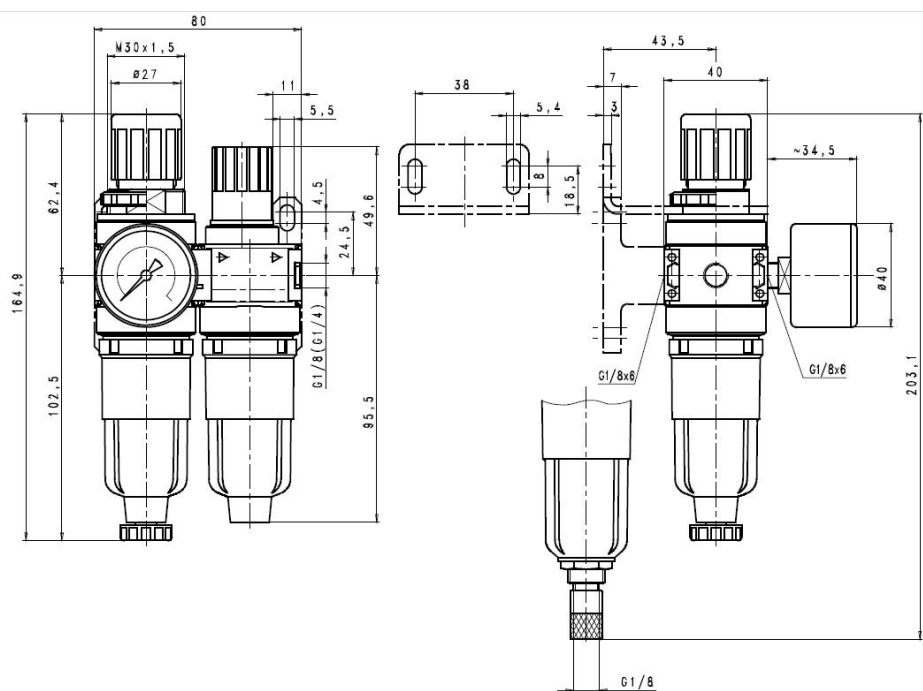
polavtomatski izpustni ventil
