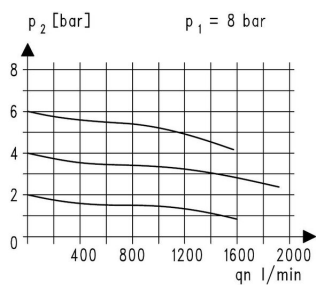
Durchflussdiagramm
