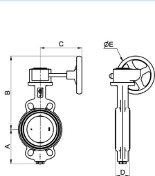
Zwischenflanschausführung
