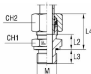
s řezným kroužkem B4
