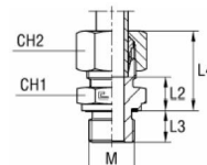
s řezným kroužkem B3
