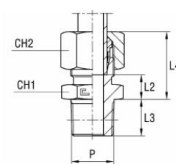
-val/-vel B3-vágógyűrűvel
