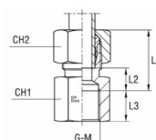
mit B3-Schneidring
