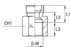
Grundkörper
