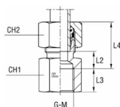
mit B4-Schneidring
