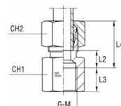
sa B3-rezni prsten
