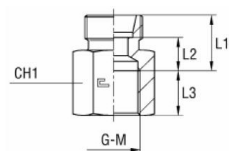
Osnovno telo
