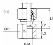
sa B4-rezni prsten
