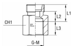
Osnovno ohišje
