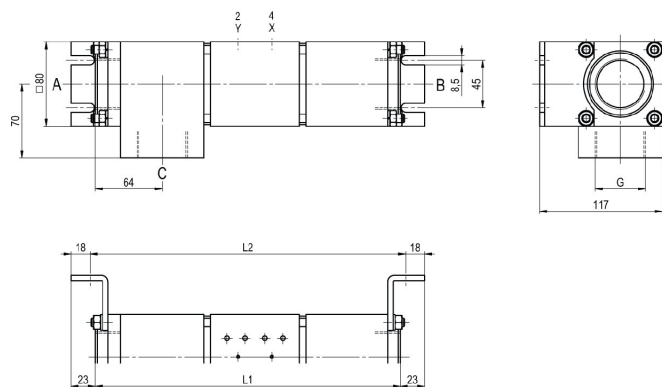
CVTV3-40 Funkció NC
