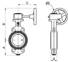
Zwischenflanschausführung
