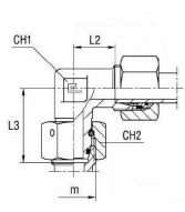
mit B4-Schneidring
