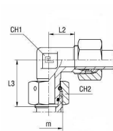
mit B3-Schneidring
