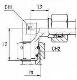
-val/-vel B4-vágógyűrűvel
