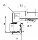
-val/-vel B3-vágógyűrűvel
