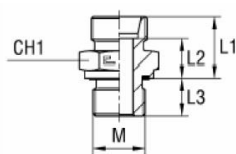
Grundkörper
