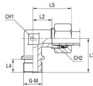
mit B4-Schneidring
