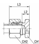
s řezným kroužkem B3
