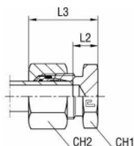
s řezným kroužkem B4
