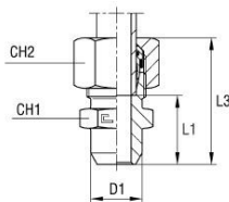
mit B4-Schneidring
