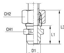
mit B3-Schneidring
