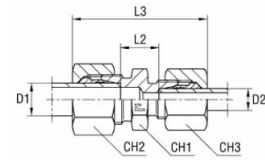
mit B3-Schneidring
