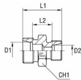
Grundkörper
