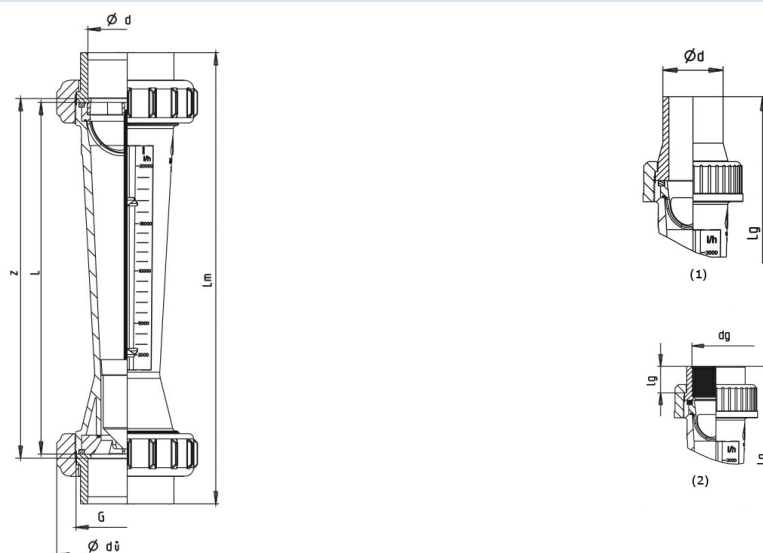
(1)...Šroubení se svařovacím nátrubkem, (2)...Šroubení se závitovou spojkou
