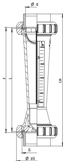
(1)...Verschraubung mit Schweißstutzen, (2)...Verschraubung mit Gewindemuffe
