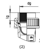
(1)...Verschraubung mit Schweißstutzen, (2)...Verschraubung mit Gewindemuffe
