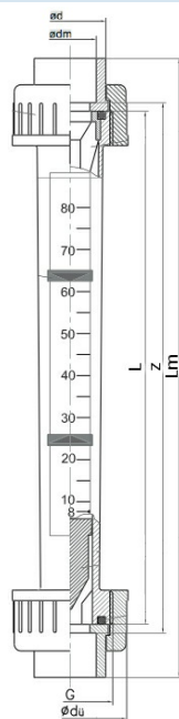
(1)...Złączka z króćcem do spawania, (2)...Złączka z mufą gwintowaną
