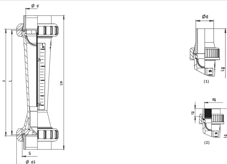
(1)...Złączka z króćcem do spawania, (2)...Złączka z mufą gwintowaną
