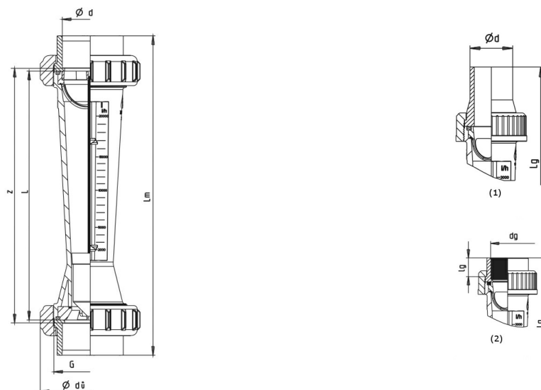
(1)...Priključak sa nastavkom za zavarivanje, (2)...Priključak sa navojnom čaurom
