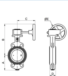
Zwischenflanschausführung
