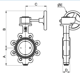
Abflanschausführung
