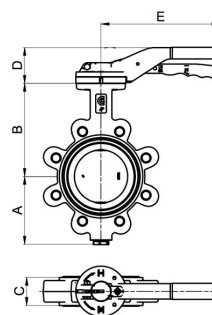
Přírubové provedení
