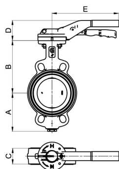
Mezipřírubové provedení
