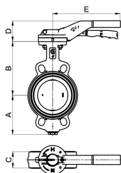
Zwischenflanschführung
