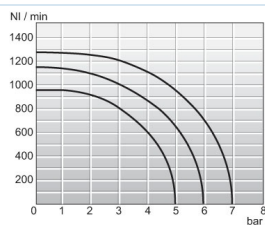
Átfolyási diagramm 1/8"
