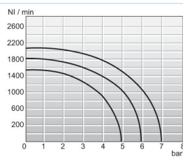
Átfolyási diagramm 1/4"
