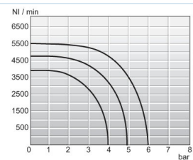
Átfolyási diagramm 1/2"
