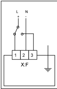
Sterowanie 3-punktowe
