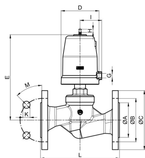
Opruga zatvara se, Tip SE24, SE25, SE33
