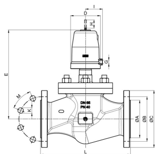
Opruga zatvara se, Tip SE24, SE25, SE33
