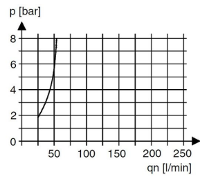
Öler-Ansprechgrenze
