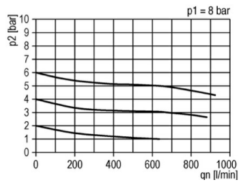
Wykres przepływu
