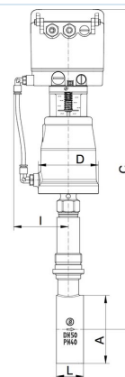
digitální polohový regulátor Typ 8049
