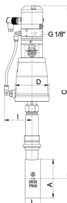
Regulator położenia I/P Typ 8047
