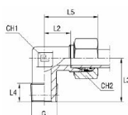
mit B4-Schneidring
