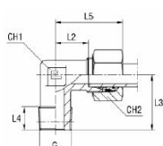
z pierścieniem tnącym B4
