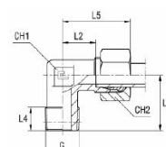
z pierścieniem zacinającym B3
