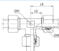
z pierścieniem tnącym B4
