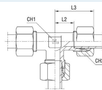
z pierścieniem zacinającym B3
