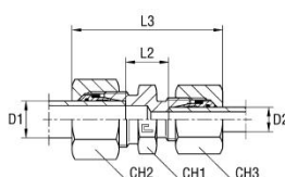
-val/-vel B4-vágógyűrűvel
