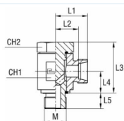
Základní těleso
