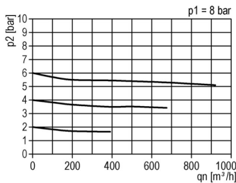
Průtokový diagramm
