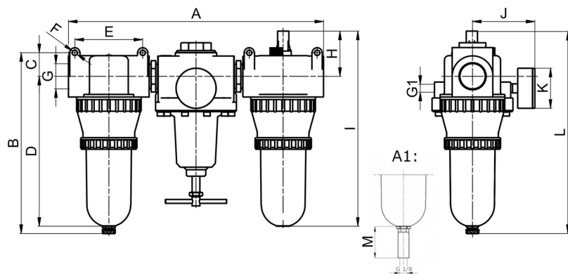
A1: automatikus leeresztőszelep
