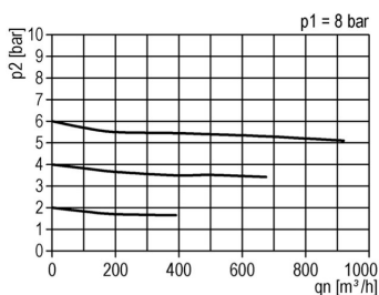
Átfolyási diagram
