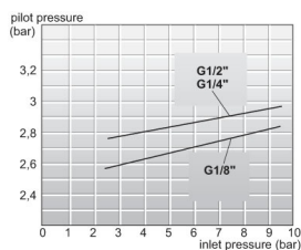
Acționare pneumatic/arcă
