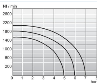
Flödesdiagramm 1/4"
