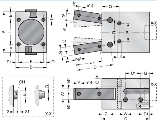
Versio läpimenevä männänvarsi
