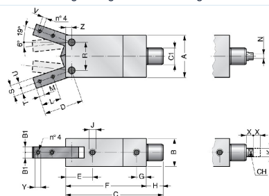
Version genomgående kolvstång:
