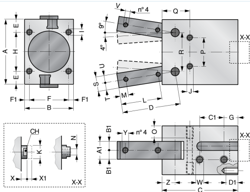
Version genomgående kolvstång
