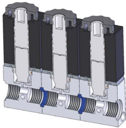
Montage des joints toriques
