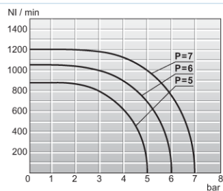
Διάγραμμα ροής 1/8"
