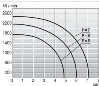
Διάγραμμα ροής 1/4"
