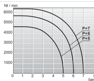
Διάγραμμα ροής 1/2"
