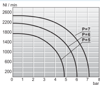
Strømningsdiagramm 1/4"
